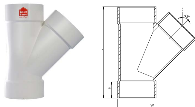
Tee 45°
