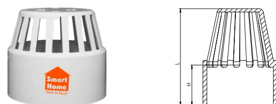
Air Vent
